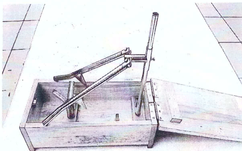
(ตัวธรรมดา) ภาพที่ 1 อุปกรณ์สำหรับปอกเปลือกทุเรียนแบบ Knock Down (กึ่งกลาง ขนาด 16 pt.) (ตัวหนา)
